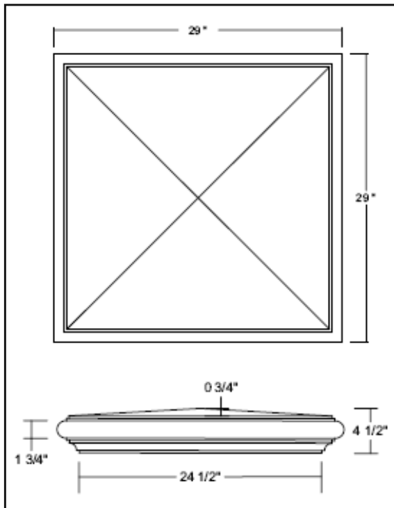
Pier Cap
